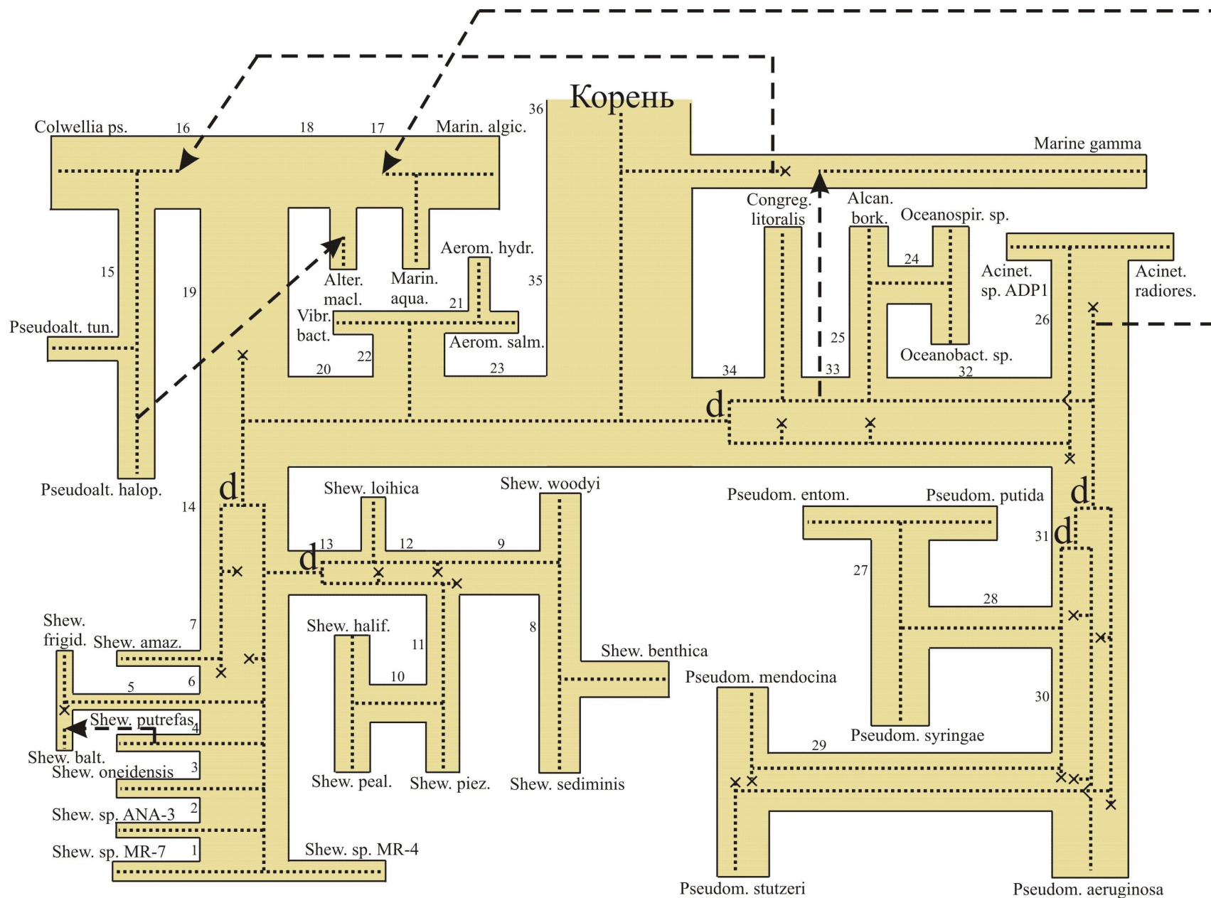
Рисунок 4. Вложение дерева G генов pro в дерево видов S , показанное на рис. 1. Ребра («трубы») дерева S показаны цветом. Дубликации обозначены буквой d , потери – крестиками, переносы – стрелками
