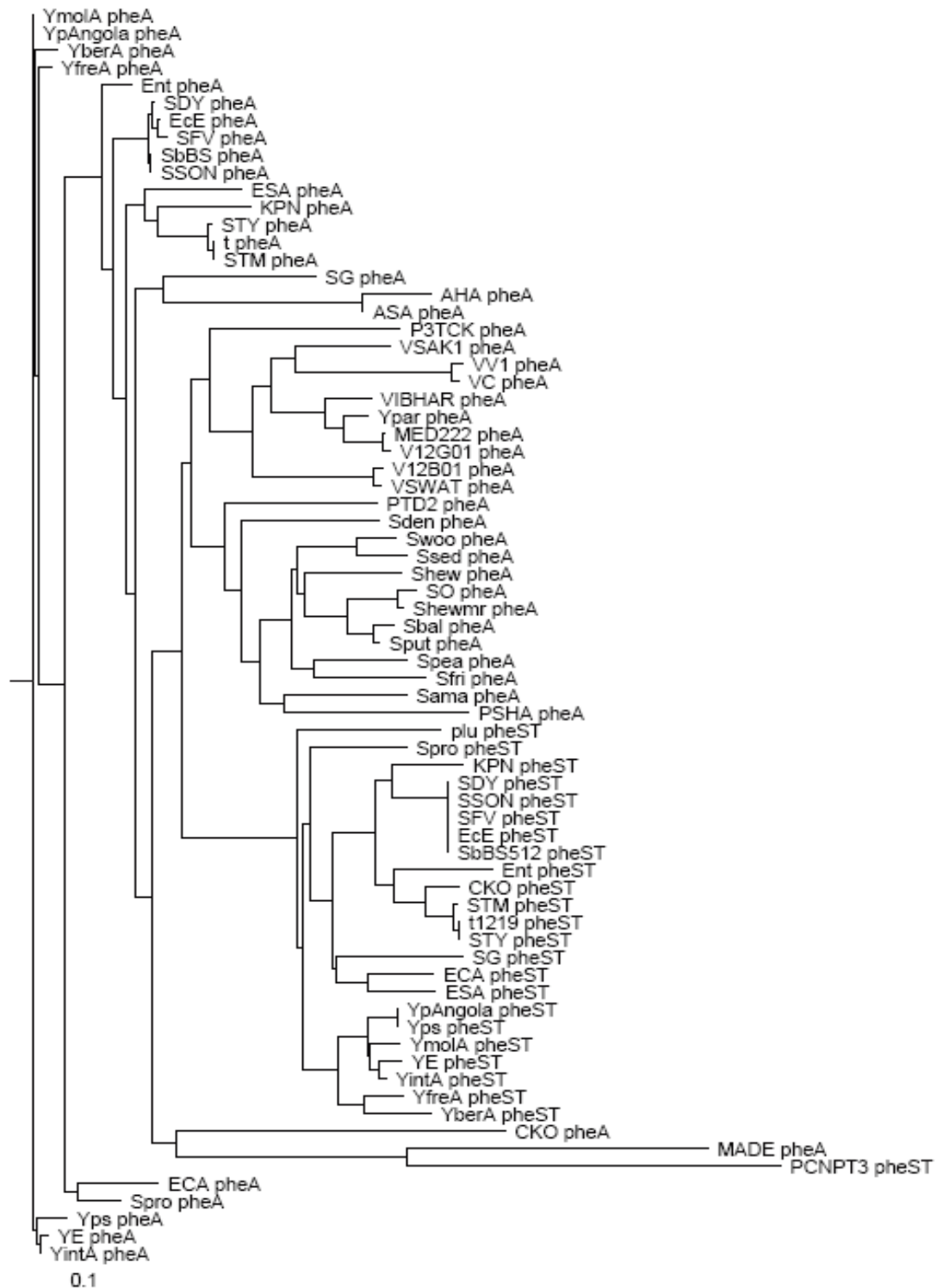
Рис. 6. Дерево регуляторных областей генов pheA и pheS у \gamma -протеобактерий. Названия видов и их сокращения приведены в таблице 2.
